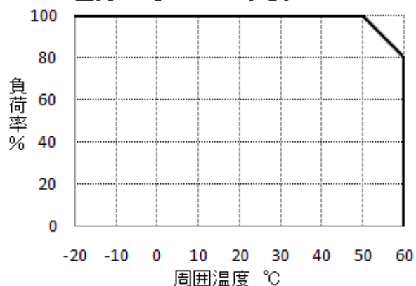
出力デレーティング表
