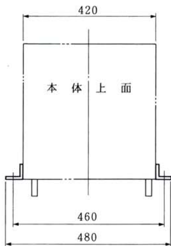
付属ラック取付金具を使用した場合の寸法
